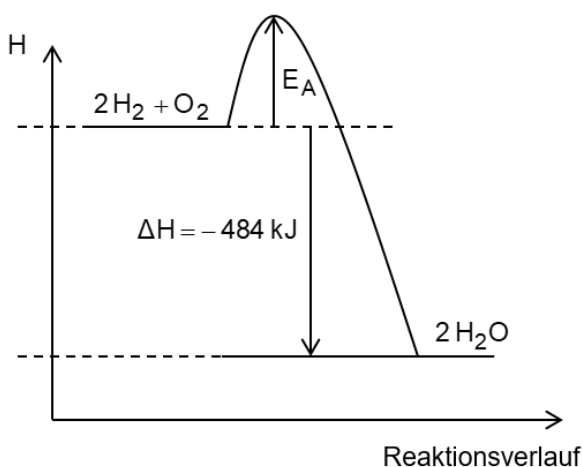
Enthalpieverlaufsdigramm
